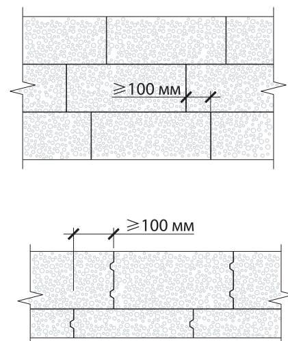
Рис. 4.4. Перевязка кладки
